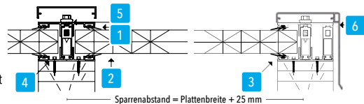
Verbindungsprofil
