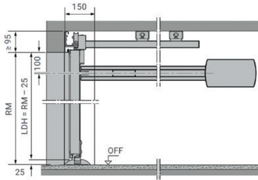
Antrieb Wandmontage
