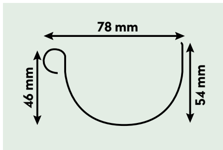
Kunststoff-Dachrinne Typ 250
