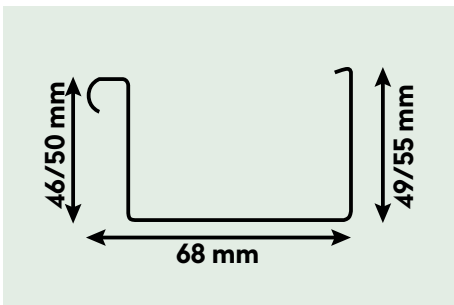
Kunststoff-Dachrinne Typ 200
