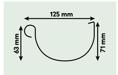
Kunststoff-Dachrinne Typ 300
